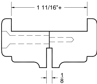
1 3/4" DOORLITE MLDG
