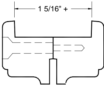
1 3/8" DOORLITE MLDG
