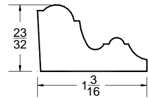
FLUSH MLDG #310
